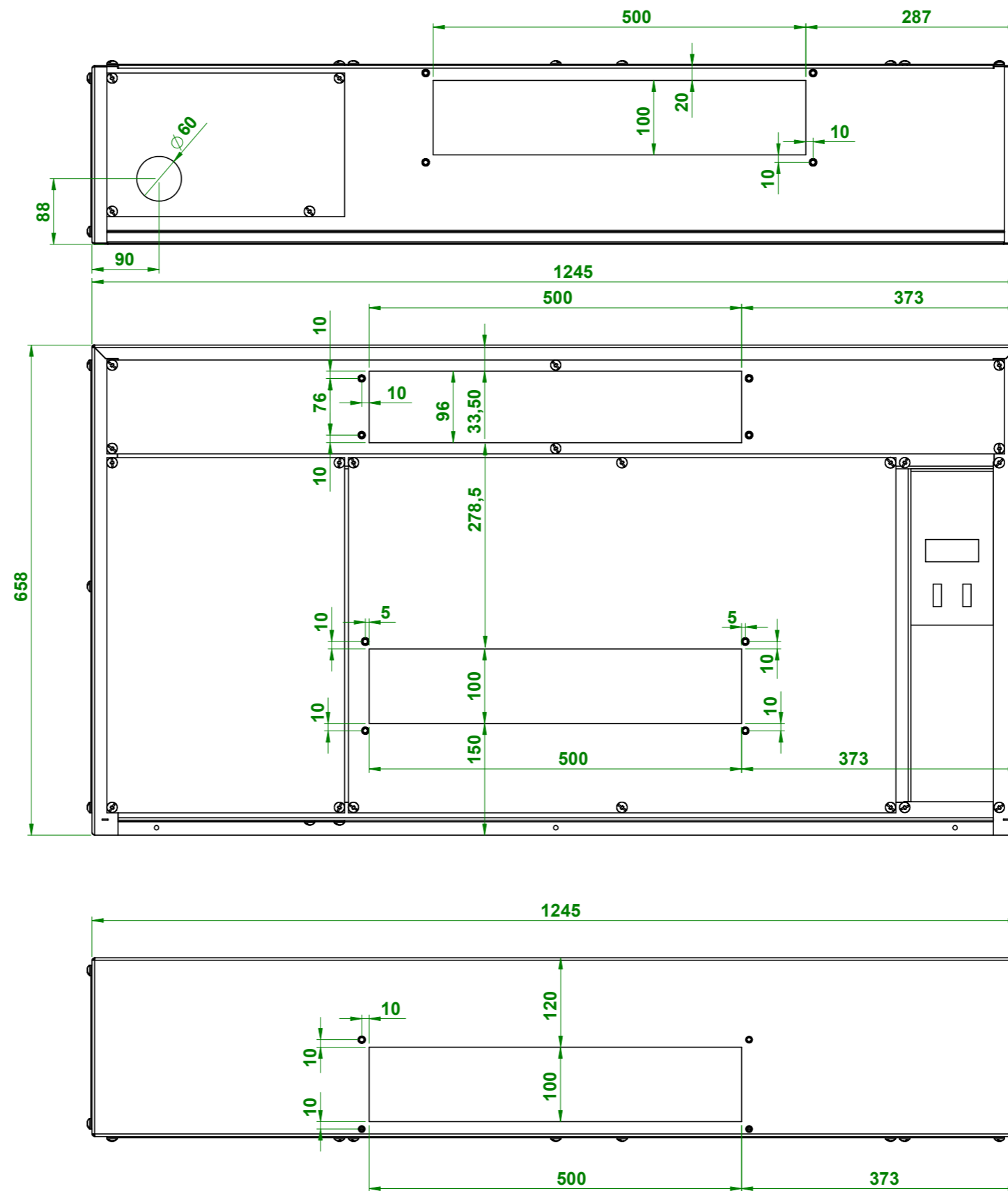
spodní pohled
